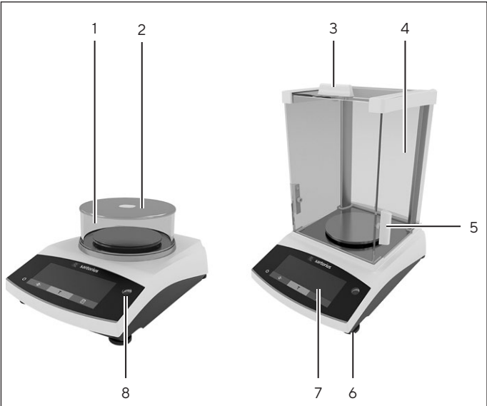
Abb. 1: Präzisionswaage mit rundem Windschutz und Analysenswaage mit Analysenwindschutz (Beispiel)
