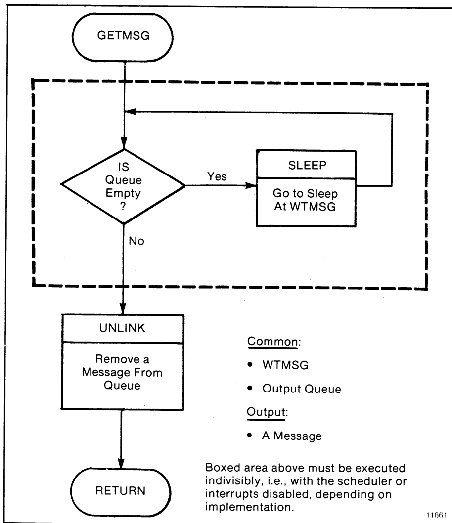
Figure D.9 — GETMSG Subroutine
