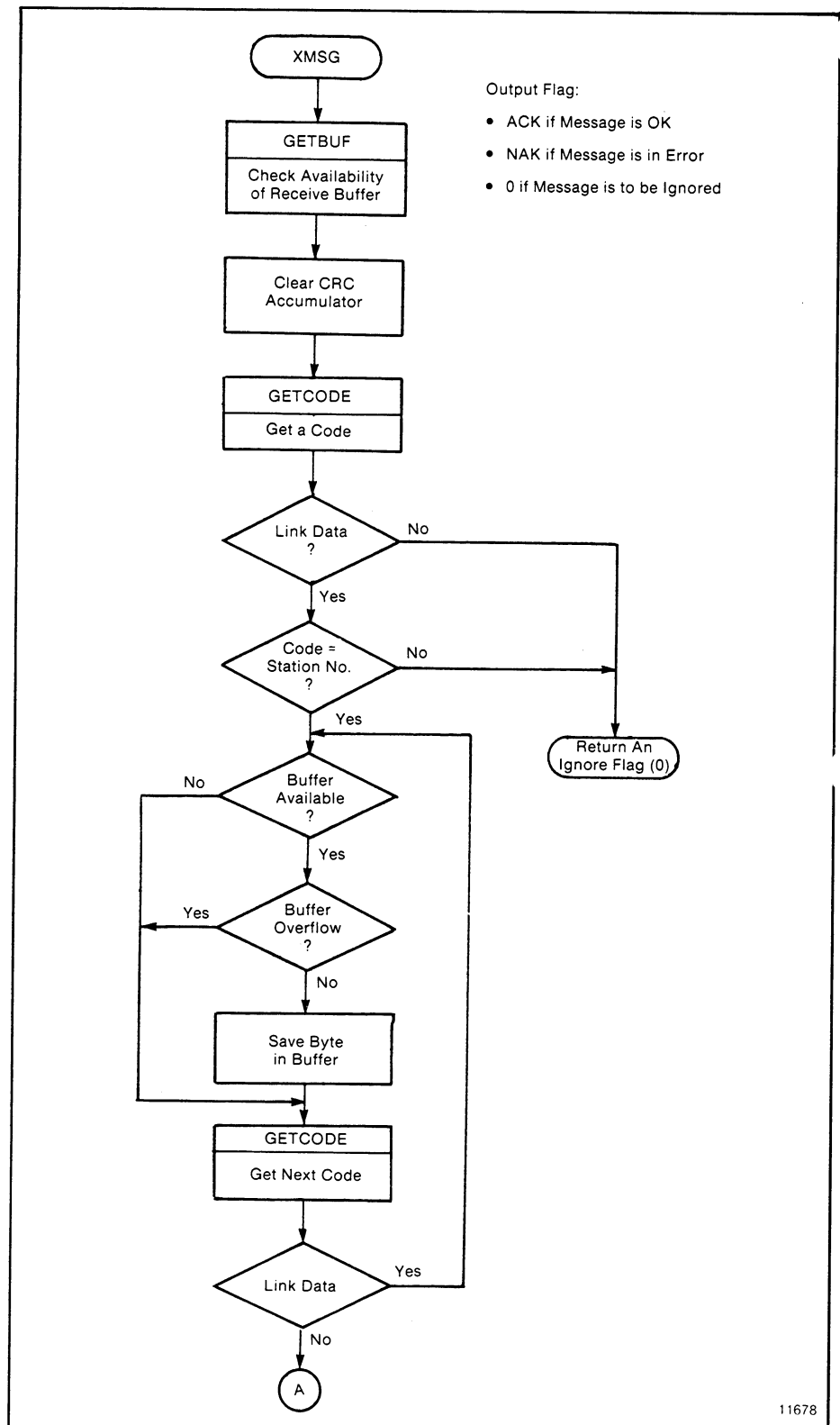
Figure D.26 — XMSG Subroutine
