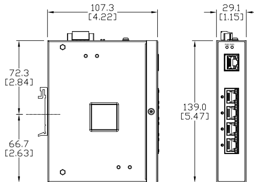
SE2-SWP5U-T SE2-SWP5UG-T
