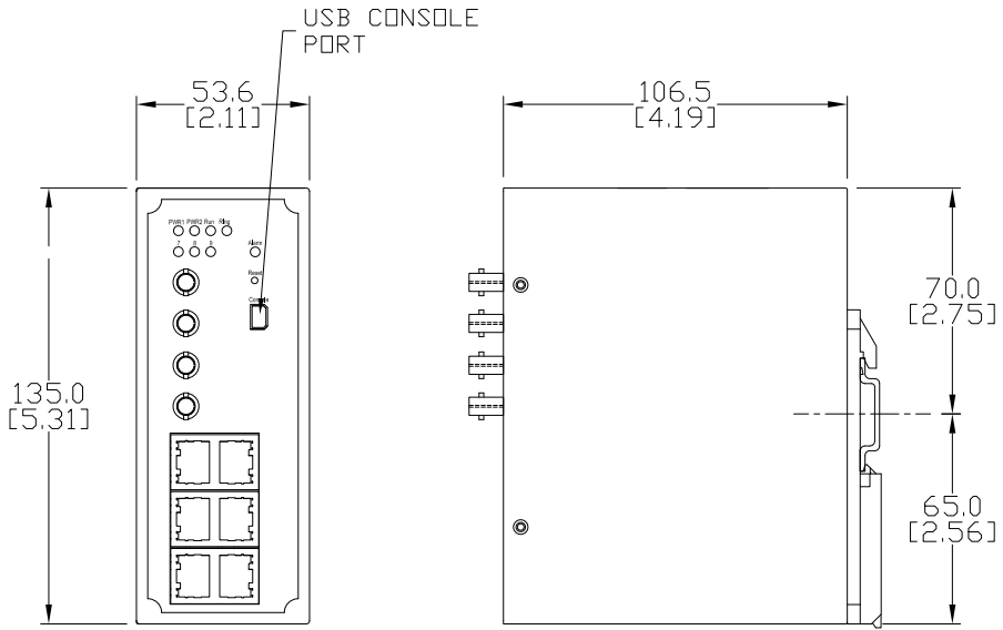
SE2-SW8M-2T1
