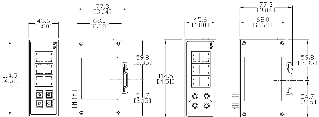
SE2-SW8U-2C1-T
