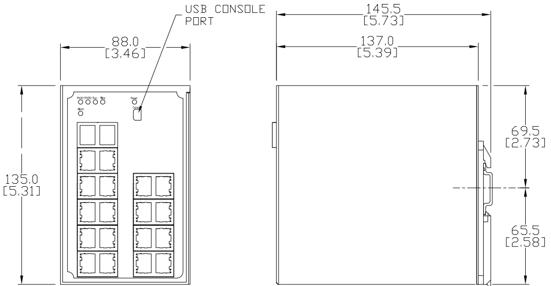
SE2-SW18MG-2P
