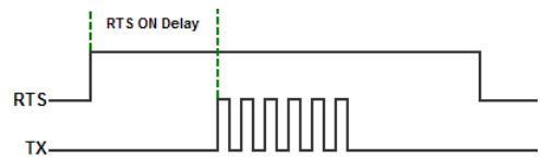
k. RTS On Delay
