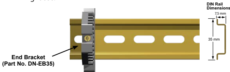
DIN Rail (Part No. DN-R35S1)
