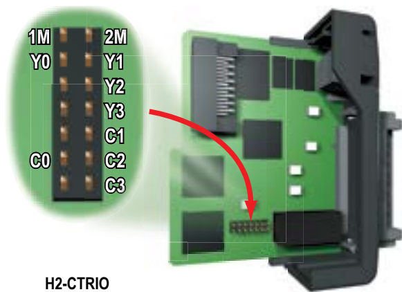
H2-CTRIO
