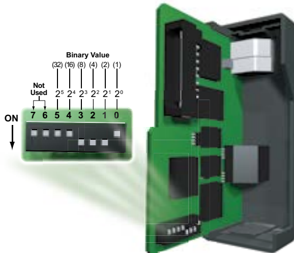
H2-ERM(100)/H2-EBC Module
